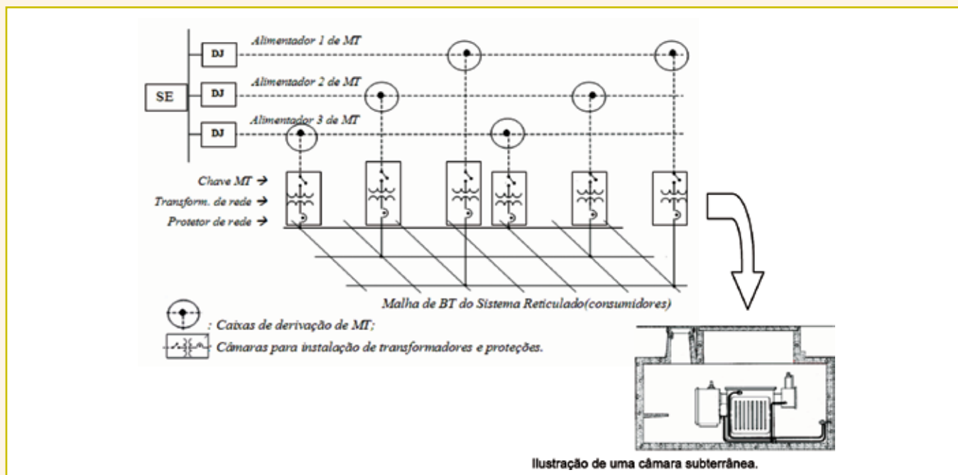
Figura 1 – Diagrama esquemático unifilar, um sistema reticulado Grid Network (reticulado malha) e ilustração de uma câmara subterrânea com o protetor de redes, o transformador e chave primária MT (da esquerda para a direita).
