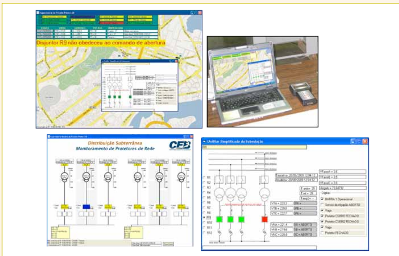
Figura 4 – Telas dos aplicativos de telemonitoramento e telecomando do protetor de rede inteligente.
