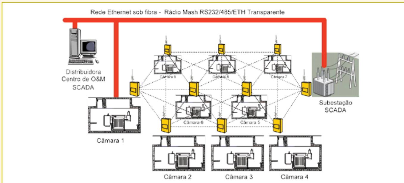
Figura 3 – Infraestrutura de comunicação por rádio mesh como uma das possibilidades para o modelo de automação híbrido nas RDS.
