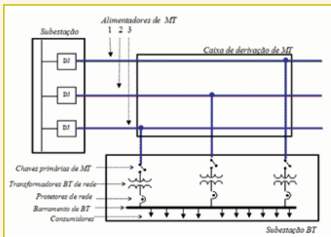
Figura 2 – Diagrama esquemático unifilar de um sistema reticulado Spot Network (reticulado exclusivo) de distribuição.
