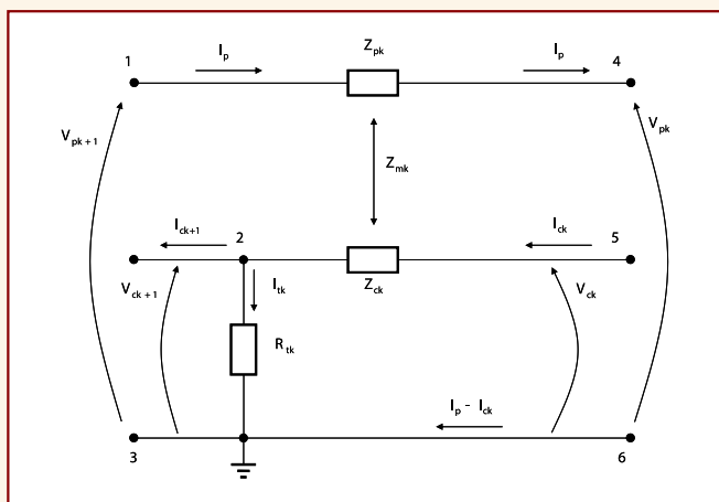
Figura 4 — Modelo completo de um vão de linha de transmissão ou rede de distribuição (Figura 8 da ABNT NBR 15751).
