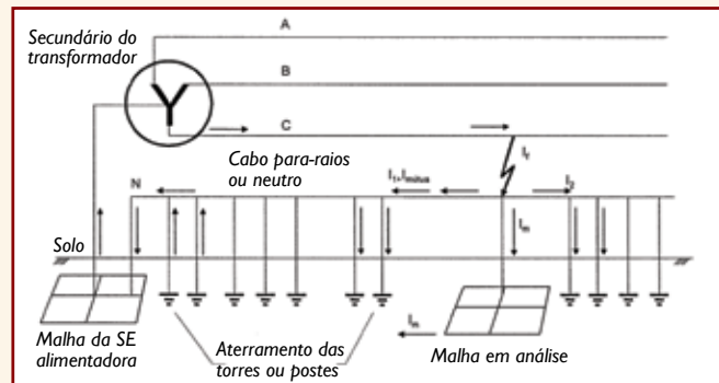
Figura 3 – Com cabo para-raios ou neutro (corresponde à Figura 7b da ABNT NBR 15751). Além das correntes já vistas também são mostradas as correntes que fluem pelo circuito formado pelos cabos para-raios e torres da linha de transmissão.
