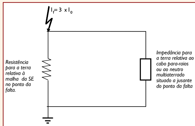
Figura 6 – Circuito do Z_{eq} da Figura 5 (Figura 10 da ABNT NBR 15751).
