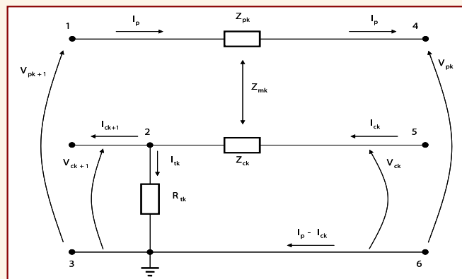
Figura 5 – Circuito elétrico para cálculo da corrente de malha considerando o sistema de potência da Figura 2 (Figura 9 da ABNT NBR 15751).
