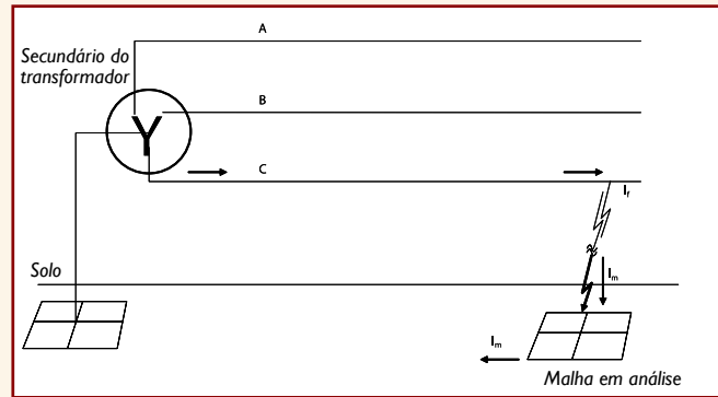
Figura 2 – Sem cabo para-raios ou neutro (corresponde à Figura 7a da ABNT NBR 15751). A corrente I_f flui integralmente do eletrodo para o solo, então I_m = I_f
