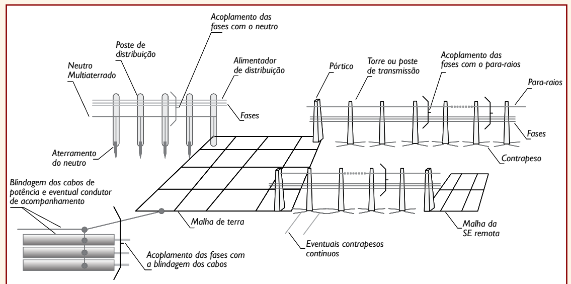
Figura 1 – Principais elementos físicos a serem considerados em cálculos e simulações para o dimensionamento de uma malha de terra.
